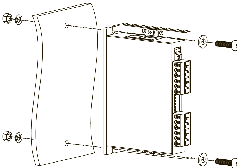
Рисунок 5.3 – Монтаж прибора
