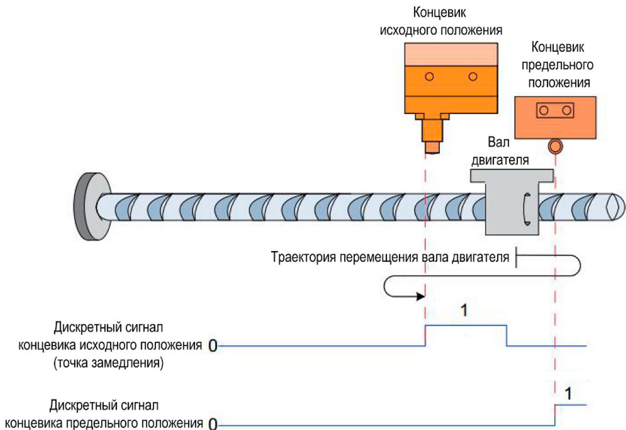
Рисунок 3.3 – Алгоритм возврата в исходную позицию с использованием сигнала концевика исходного положения при начальном условии 3
