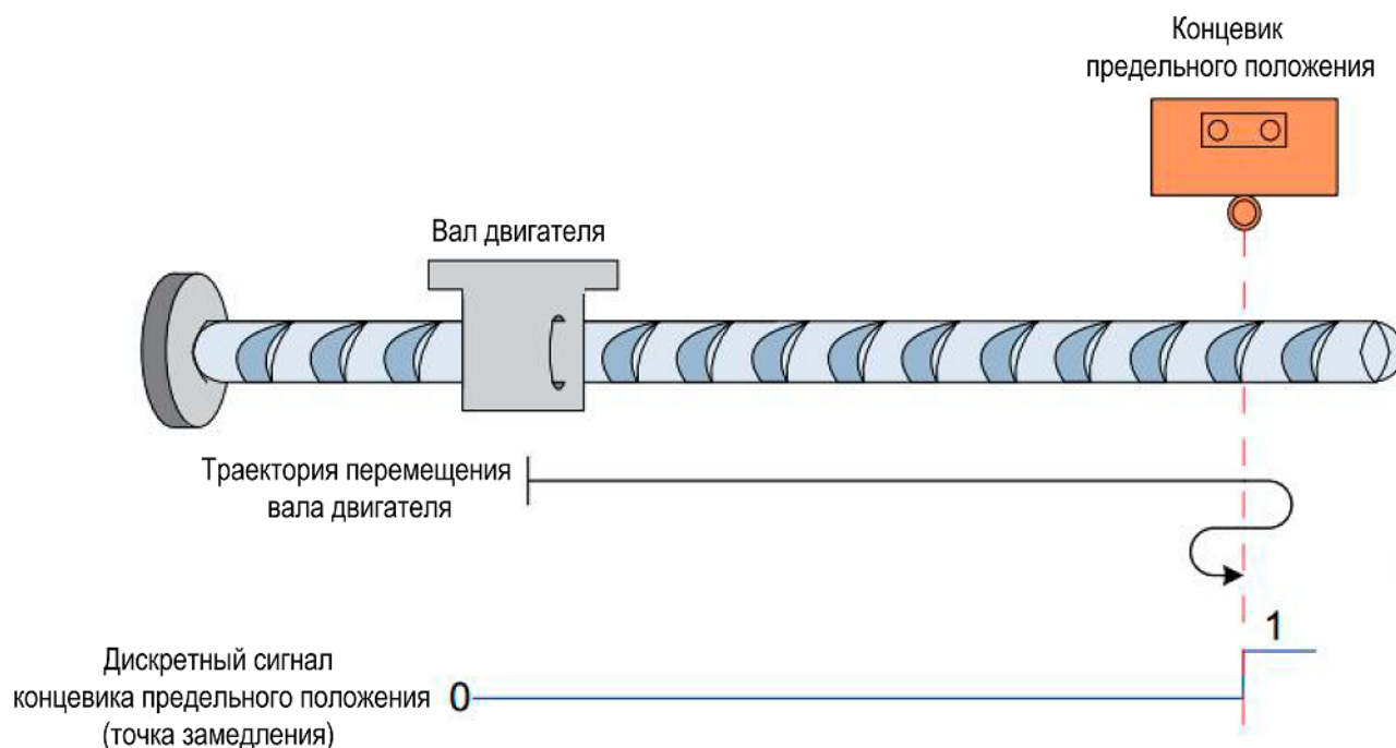
Рисунок 3.4 – Алгоритм возврата в исходную позицию с использованием концевика предельного положения при начальном условии 1
