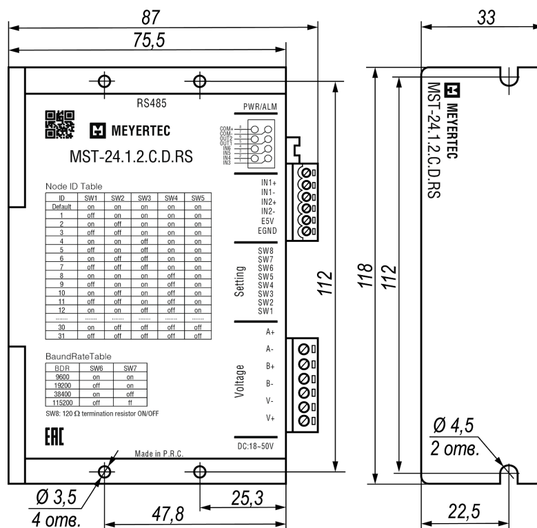
Рисунок 5.2 – Габаритные и установочные размеры прибора
