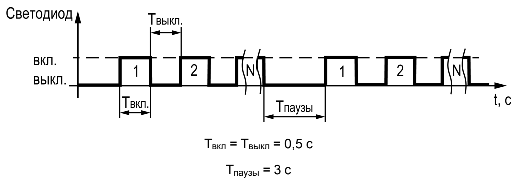
Рисунок 7.2 – Диаграмма индикации критических и не критических аварий
