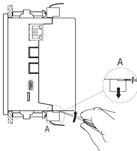
Рисунок 5.3 – Отсоединение съемных частей клемм
