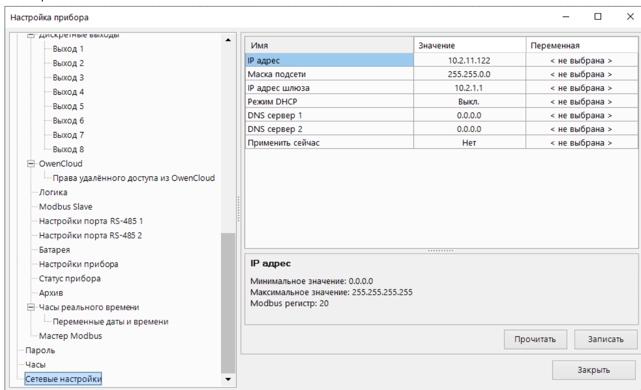
Рисунок 4.16 – Настройки параметров Ethernet
