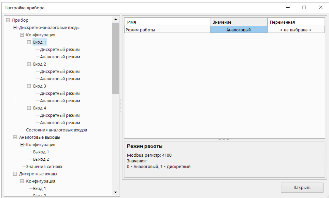
Рисунок 4.1 – Настройка режима работы входа
