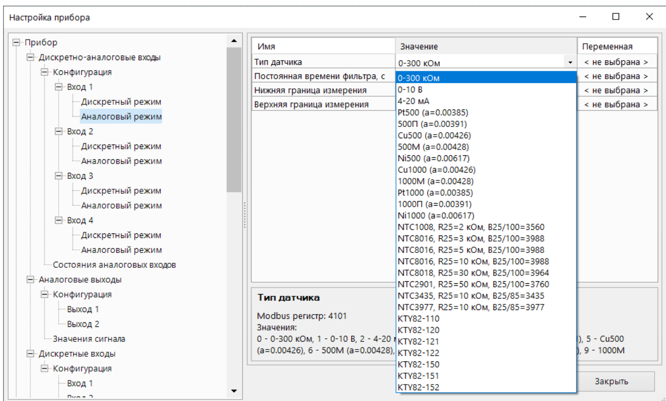
Рисунок 4.2 – Меню настройки аналогового режима входа
