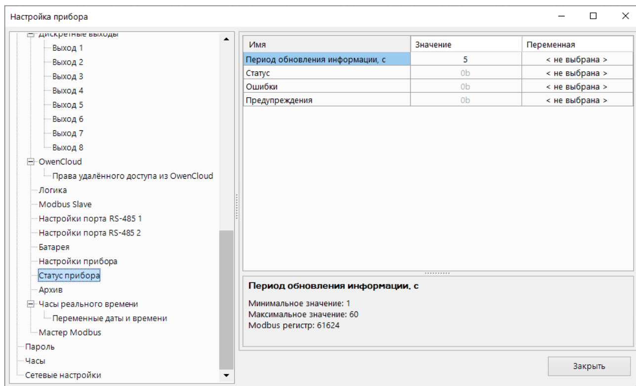
Рисунок 4.33 – Параметры статуса прибора
