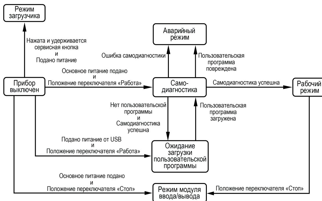
Рисунок 7.6 – Схема переходов между режимами работы
