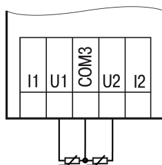
Рисунок 6.8 – Подключение ТС к аналоговому входу
