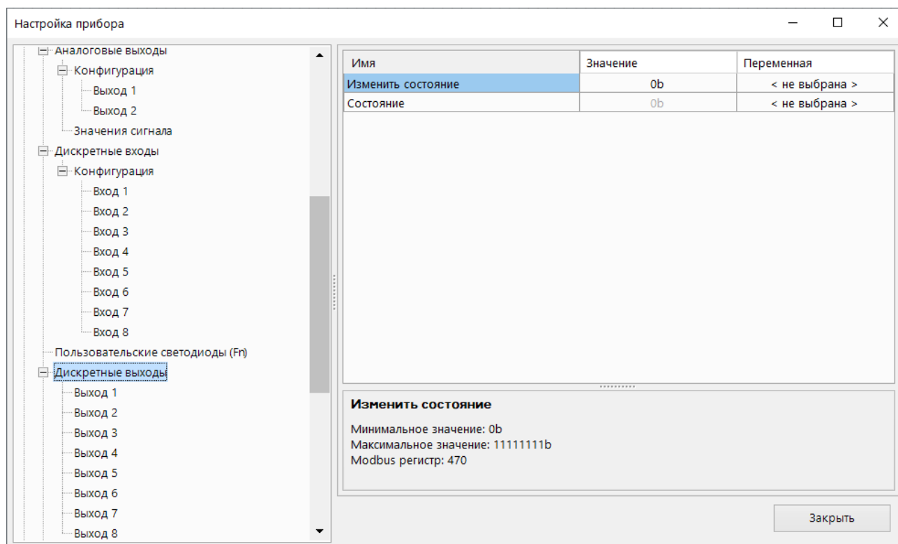
Рисунок 4.10 – Состояние дискретных выходов
