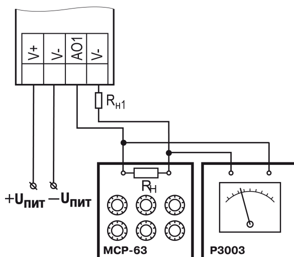
Рисунок В.3 – Схема подключения к ВЭ для юстировки сигналов типа «4...20 мА» ( R_n < 300
