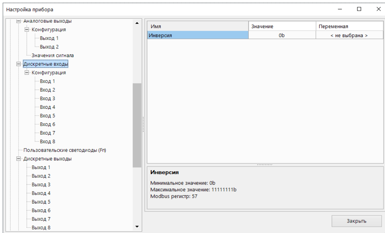
Рисунок 4.6 – Настройка инверсии дискретных входов
