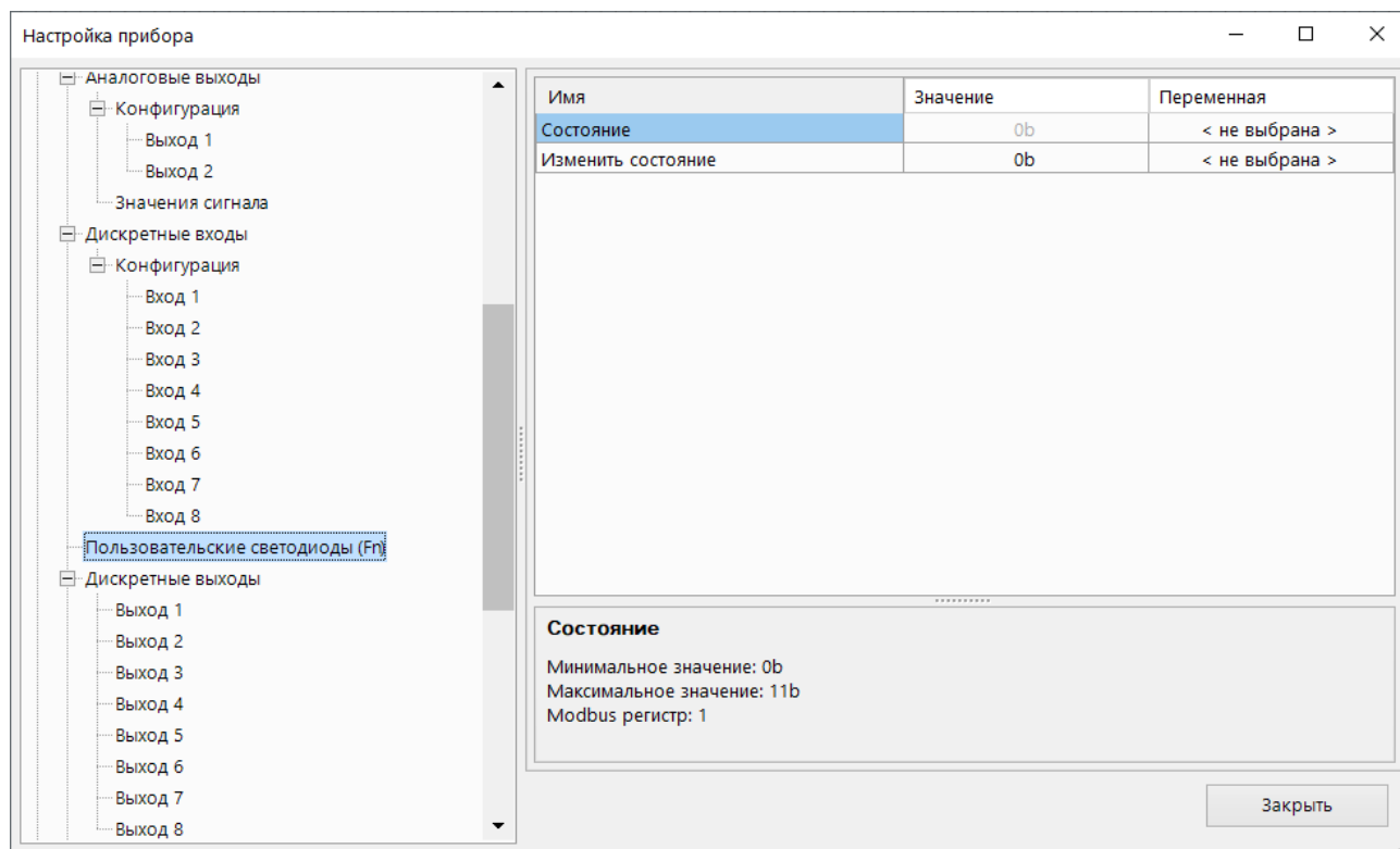
Рисунок 4.8 – Состояние программируемых светодиодов F1 и F2
